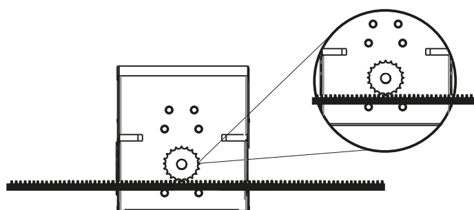
Figura 03: Fixar a cremalheira no portão, com um ponto de solda, observando que a engrenagem se encaixe na cremalheira, para que ocorra a movimentação do portão no momento que o movimentador for acionado.
